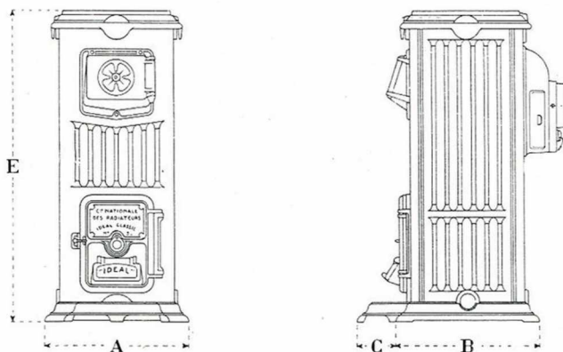
Chaudière "IDÉAL CLASSIC" vue de face et vue de profil.
