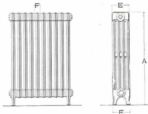
Radiateur "IDÉAL CLASSIC" n° 4, vu de face et vu de profil.
