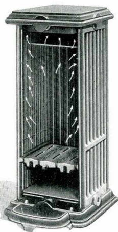
Vue intérieure de la Chaudière "IDÉAL CLASSIC", le panneau avant enlevé, montrant la grille à charbon et le cheminement des flammes qui lèchent les panneaux tubulaires contenant l'eau à chauffer.
