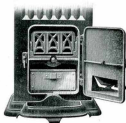
Partie inférieure de la Chaudière "IDÉAL CLASSIC" avec la porte de cendrier ouverte, montrant la grille verticale et le tiroir-cendrier.
